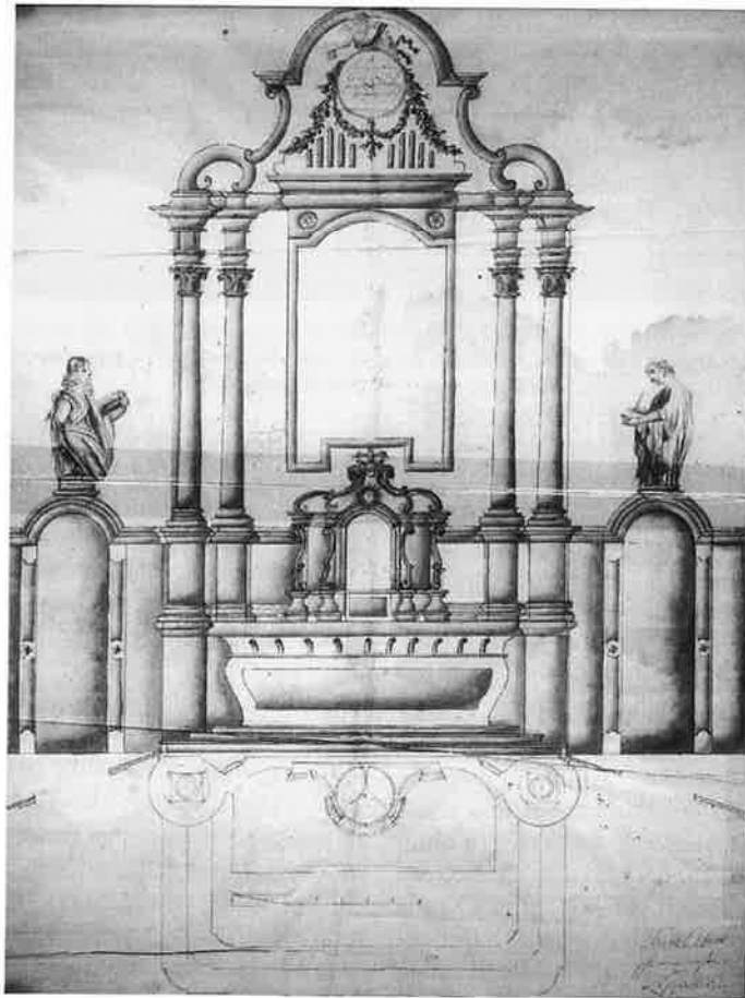
Entwurf für den Hochaltar der neuen Kirche in Kaunitz, gefertigt von dem Lippstädter Schreinermeister Franz Ebbes (ca. 1748). Die Ausführung lag bei dem Barockbildhauer Joseph Licht in Zusammenarbeit mit dem Rietberger Hofschreiner Philipp Löher.
