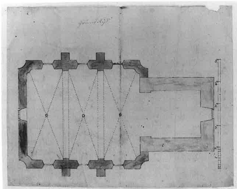
Nach diesem Grundriß entstand mit geringen Abweichungen die Kaunitzer Barockkirche.
