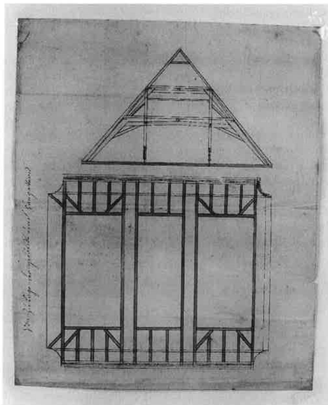
Skizze vom Dachgebälk und Hangwerk der dreijochigen Kirche. Der Entwurf ist wohl dem Zimmermeister Dieden zuzuschreiben.
